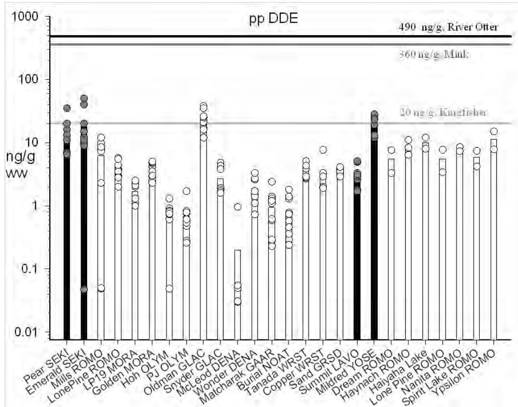
Figure 7.3 pp'DDE
